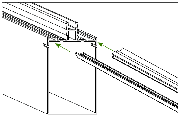
Mittelsparren
