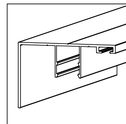
Randsparrenabdeckprofil
