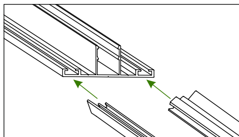
Sparrenabdeckprofile
