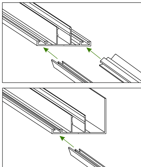
Sparrenabdeckprofile
